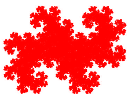
Courbe du dragon
