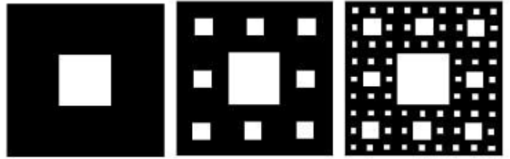
Les premières étapes de la construction du tapis de Sierpinski
