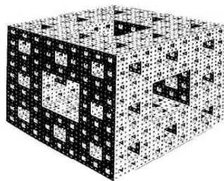
Eponge de Menger
