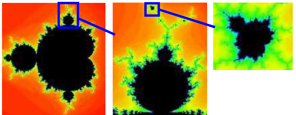
L'ensemble de Mandelbrot
