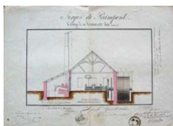
Plan des forges de Paimpont par Chéron (Stanislas Victor), Ingénieur des mines (1787-1852) Archives nationales
