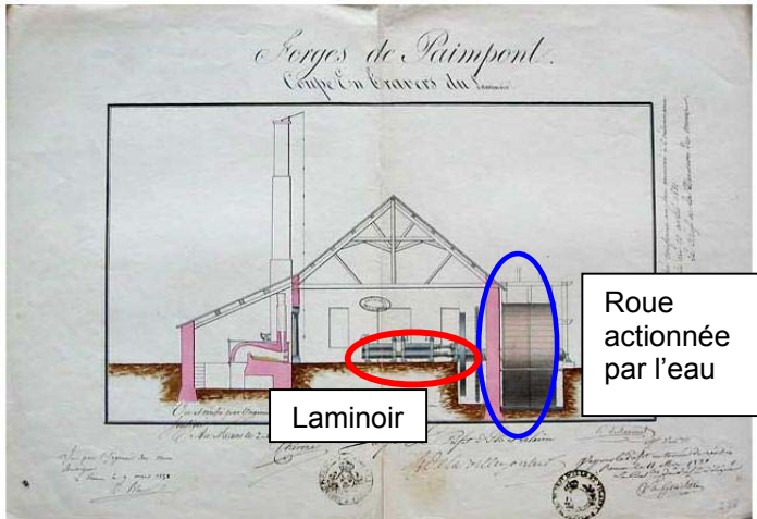
Gravure Coupe en travers du Laminatoire - Forges de Paimpont
